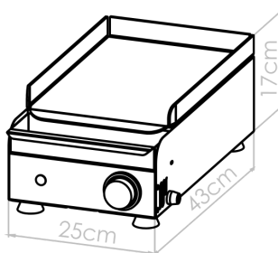
DIAGRAMA TÉCNICO · COTAS EN CM
